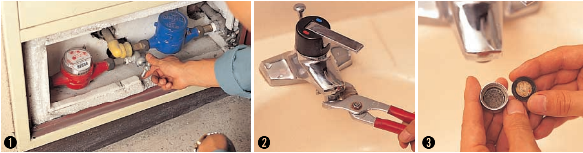
① 수도관 밑에 있는 나사를 풀어준다. ② 수도꼭지 속에 있는 그물망의 이물질 제거한다. ③ 수도꼭지를 다시 죄어준다.
